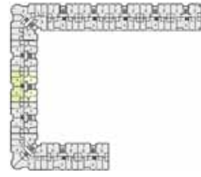
ТИПОВЫЕ ПЛАНИРОВКИ СЕКЦИИ №5. 2-5 ЭТАЖИ
